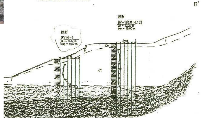
虫崎側擁壁縦断面図
